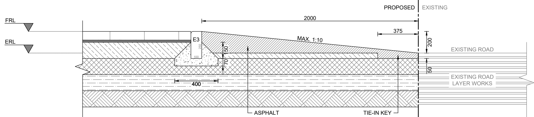
SECTION A-A SCALE 1:20
